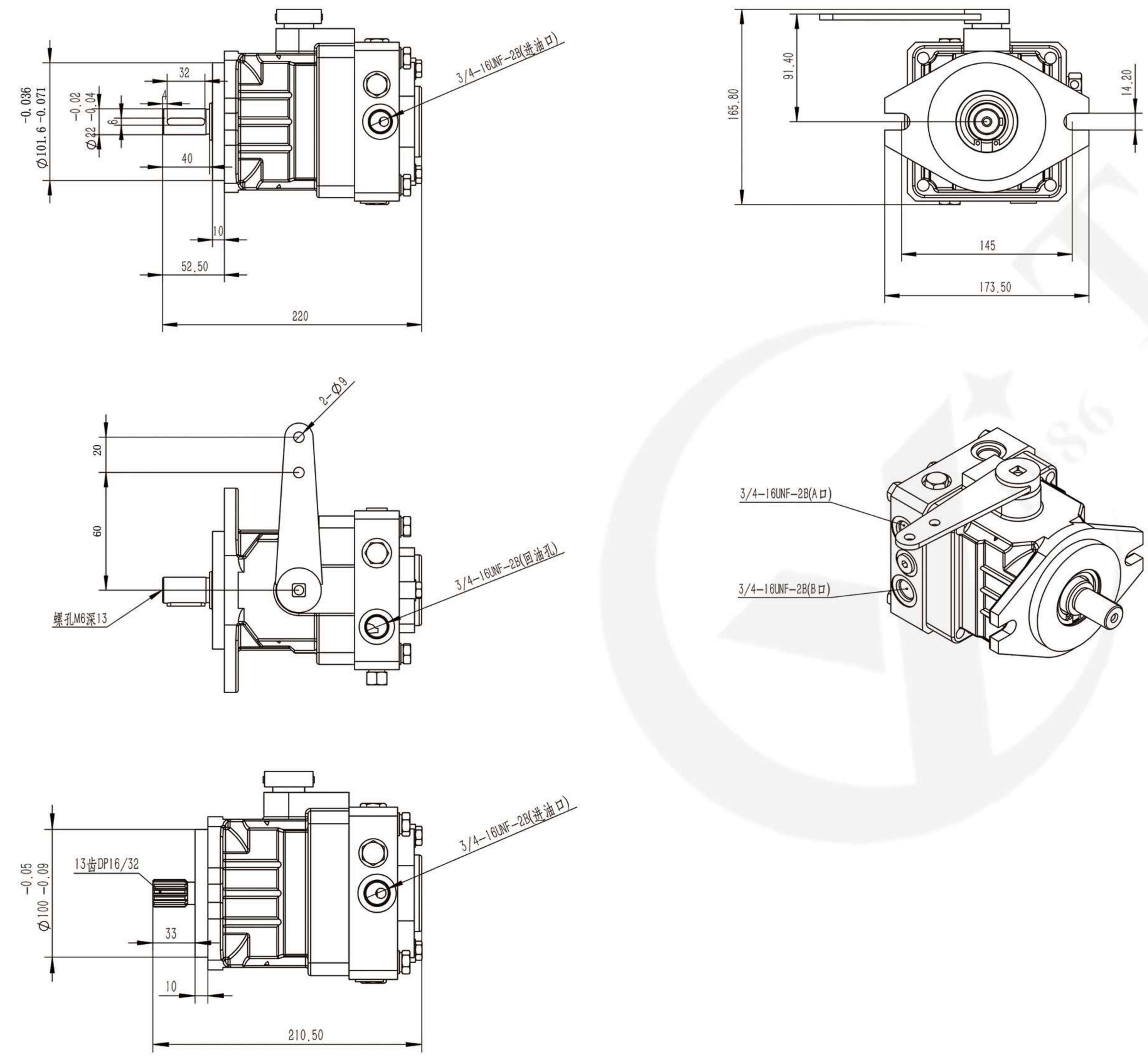
连接尺寸
