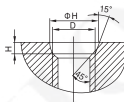
油口尺寸
