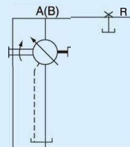
手动变量 MA Manual control
