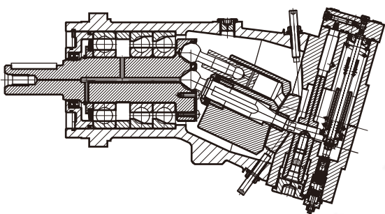
系列Series1 规格Size20-160
