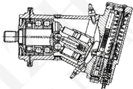
系列Series 5.1 规格Size250-500
